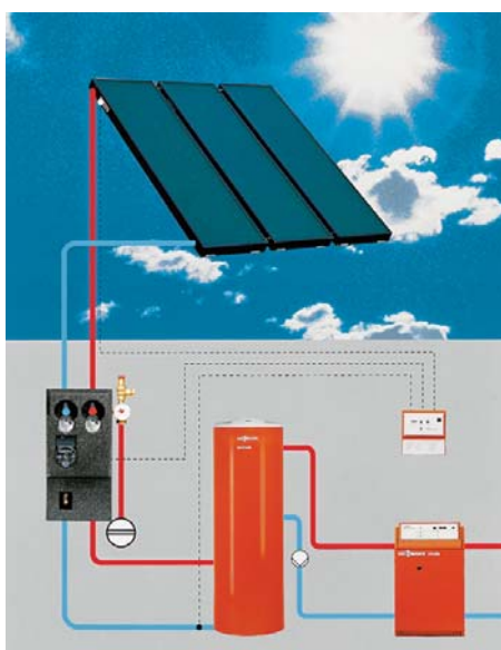
Figura 1. Componentes de una instalación solar.
