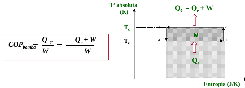
Figura 3. Ciclo Bomba de calor.
